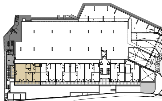
GRUNDRISS BK 01
