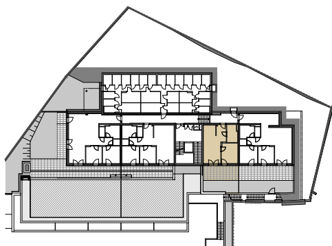
GRUNDRISS BK 04
